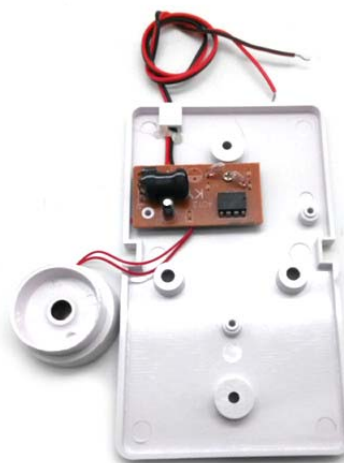
Вид устройства изнутри. Рис. 2
