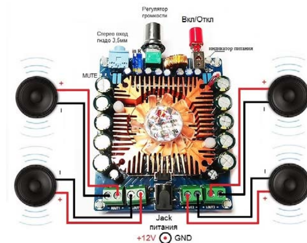
Схема подключения. Рис. 2
