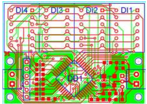
Рис. 2. Печатная плата.
