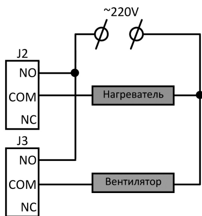
Рис. 2. Подключение нагрузки.
