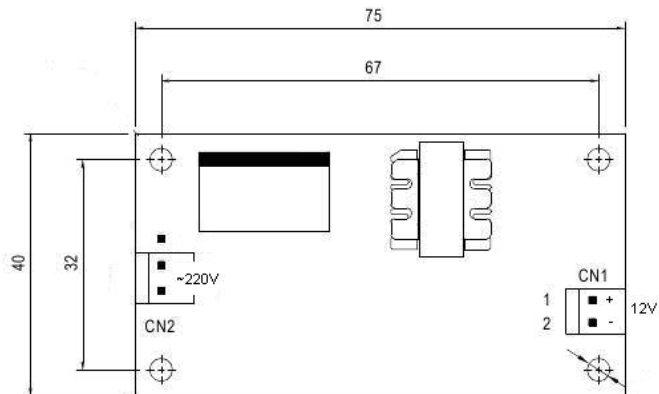
Эскиз подключения. Рис. 2
