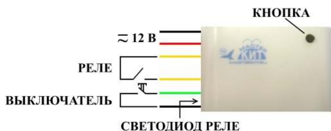
Рис. 2 Подключение устройства
