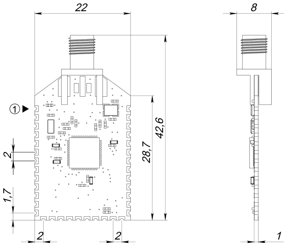
Рисунок 1. Физические размеры модуля MBee-868-3.0
