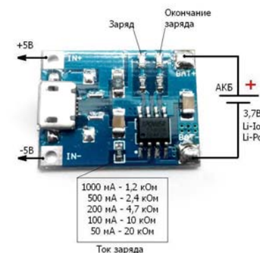
Подключение. Рис. 2
