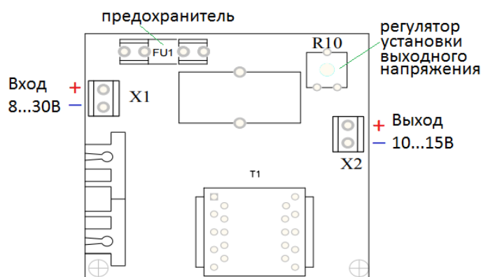
Эскиз подключения
