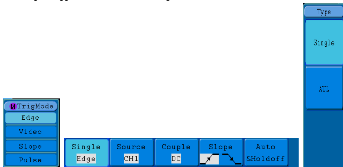
Fig. 5-17 Edge trigger menu
