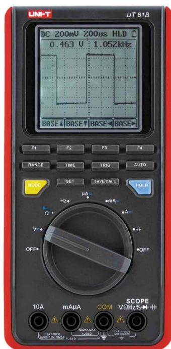
UT81B
