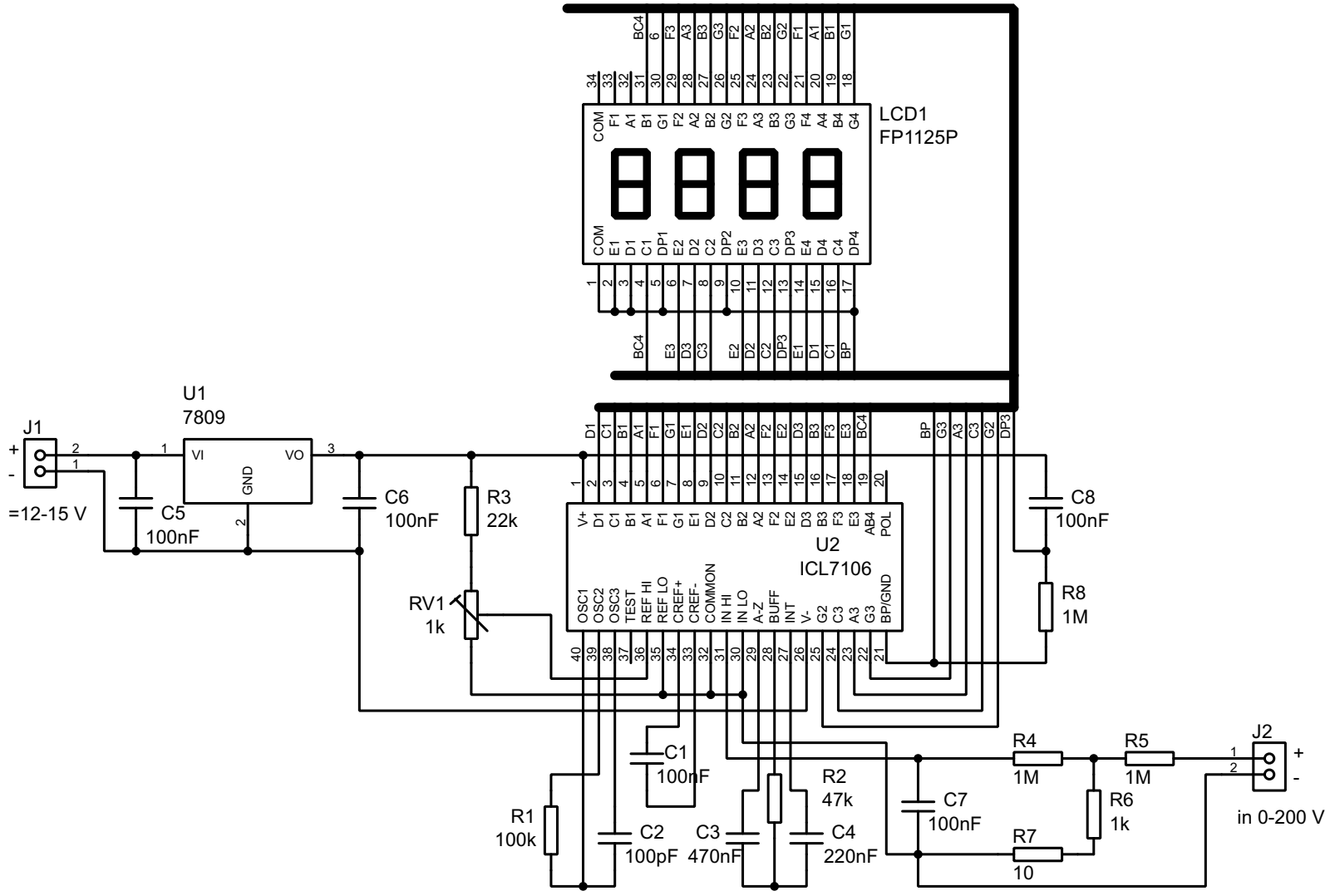
Вольтметр 0 - 200 В
